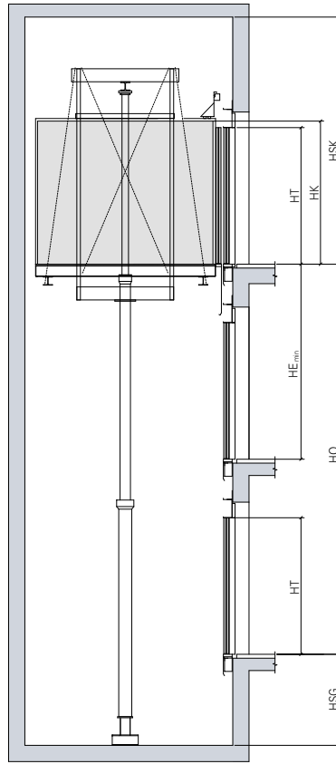
Toegang aan een zijde Tandemsysteem
