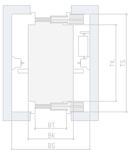
Accès de deux côtés Porte télescopique
