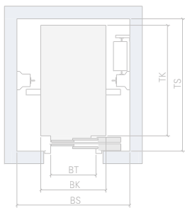
Accès d'un seul côté Porte télescopique
